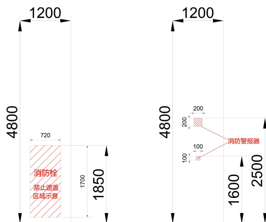
尺寸图：
