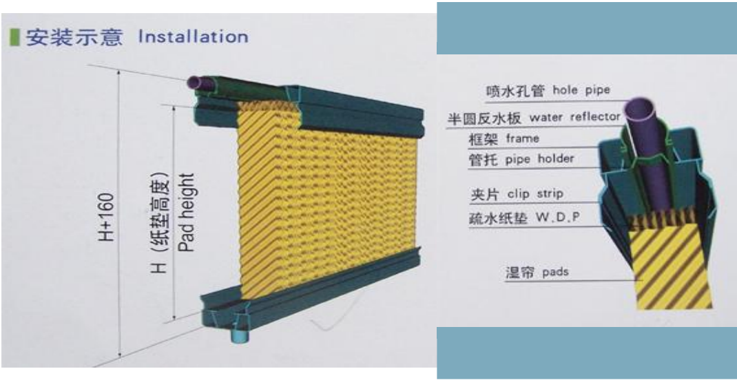
安装示意
